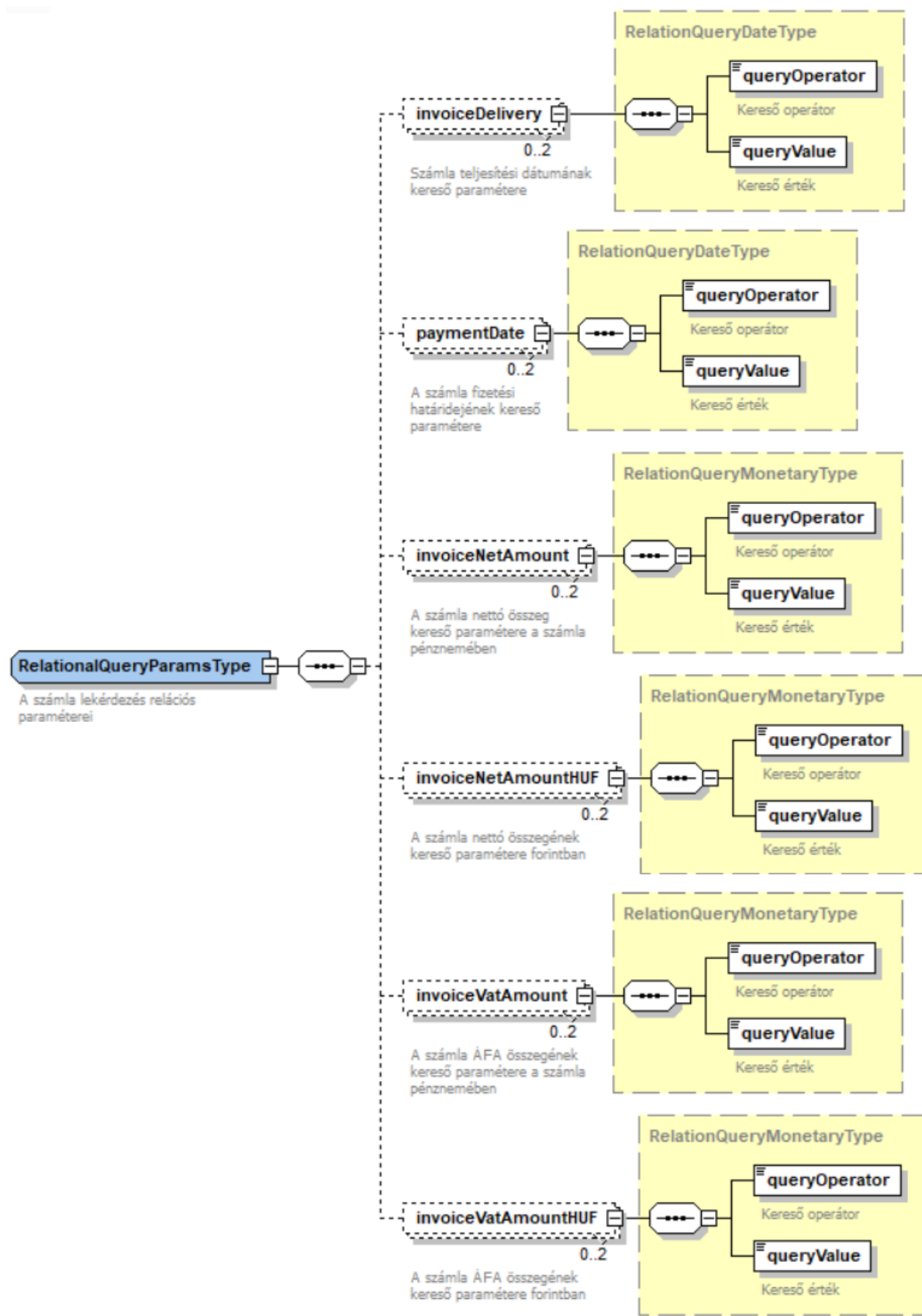
22. ábra A RelationalQueryParamsType felépítése
