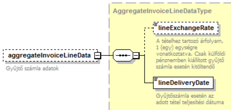
64. ábra Az AggregateInvoiceLineDataType felépítése
