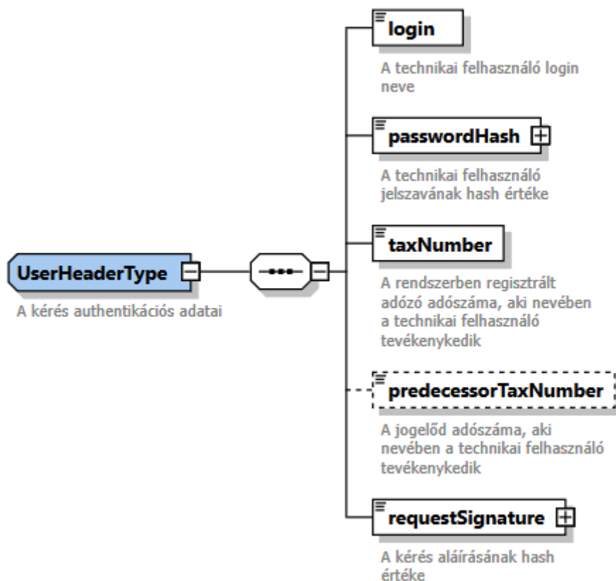
3. ábra A UserHeaderType felépítése
